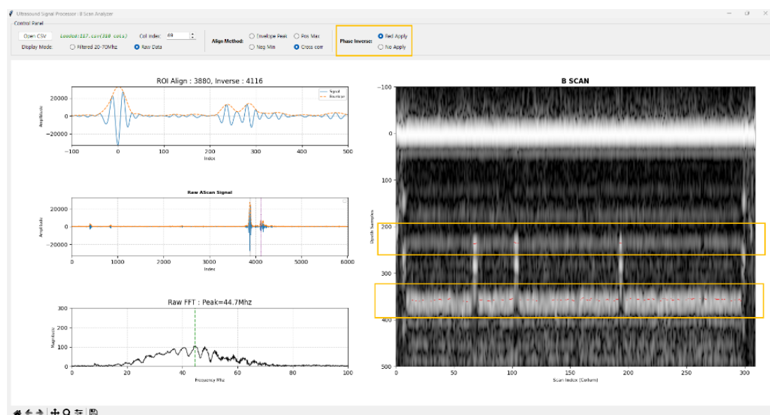
그림 8. 소프트웨어
