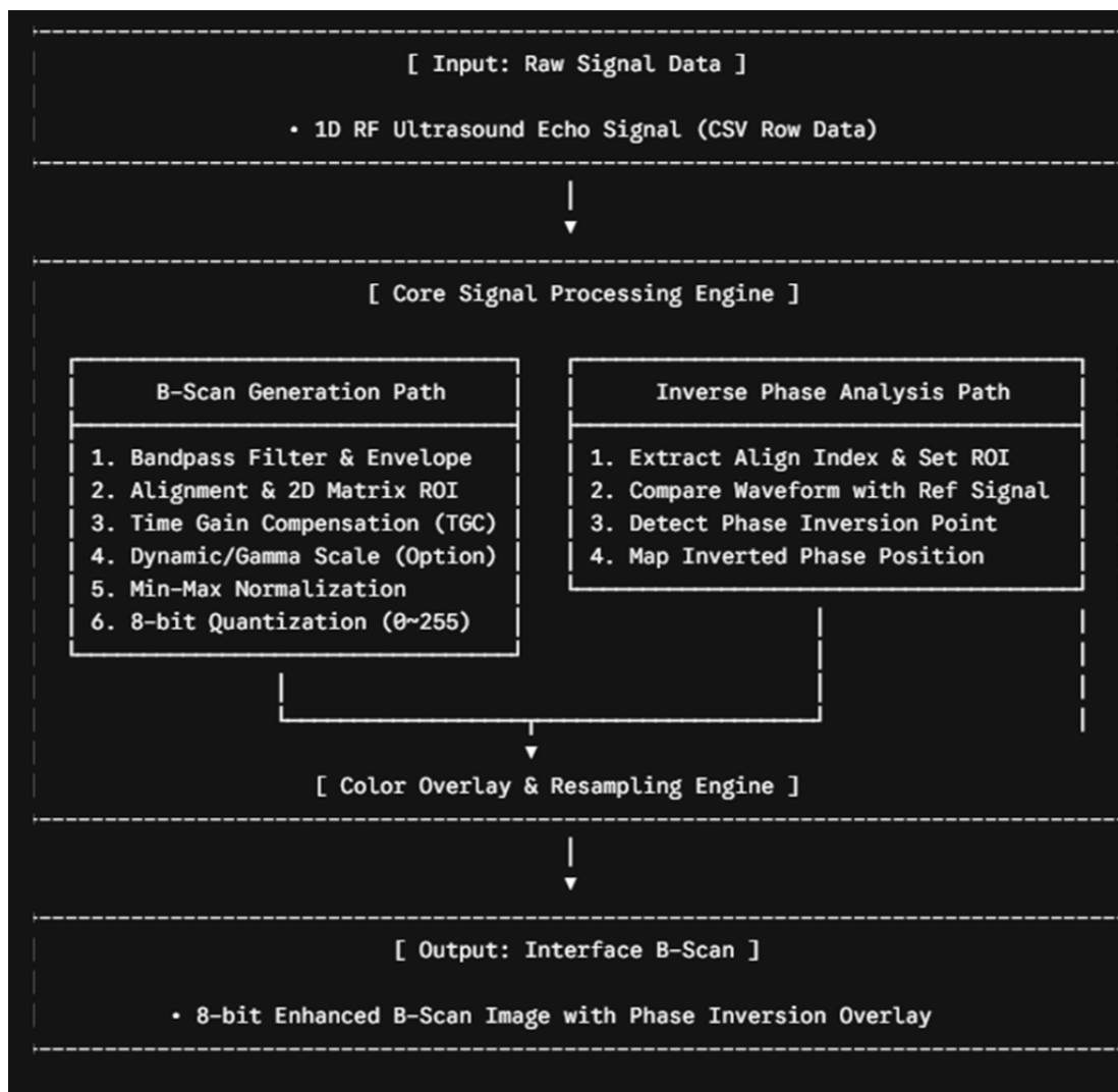
그림 7. 프로그램 내부 로직
